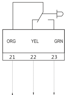
Концевые выключатели
