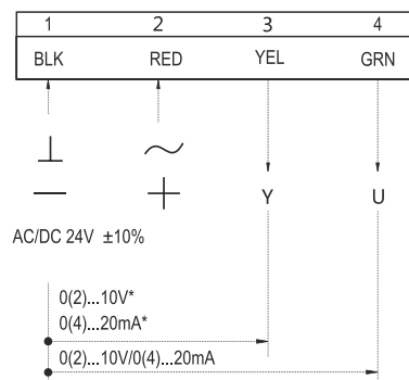
24V Привод
