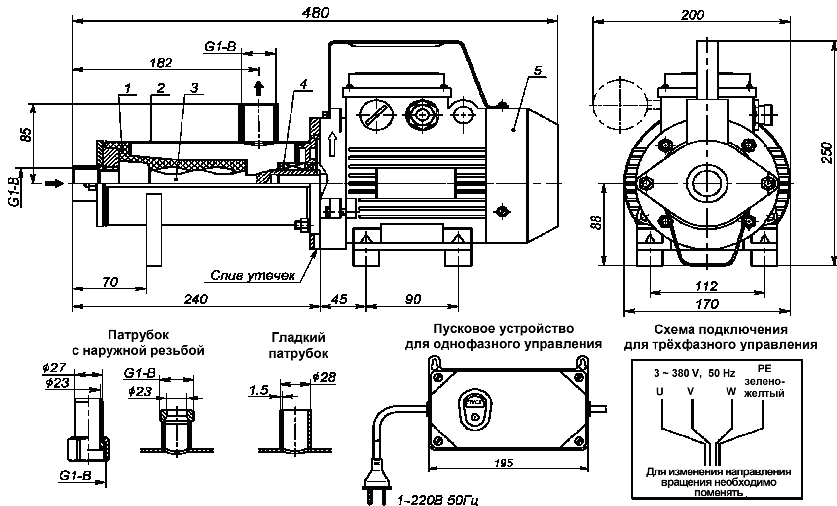
Рисунок 3 – Устройство электронасосов Бурун® CX: 0,9/4-0,25/8, 1,2/4-0,37/6, 1,8/4-0,55/4, 3,6/4-0,75/2. 1 – Обойма; 2 – Корпус насоса; 3 – Винт рабочий; 4 – Торцовое уплотнение; 5 – Электродвигатель.
