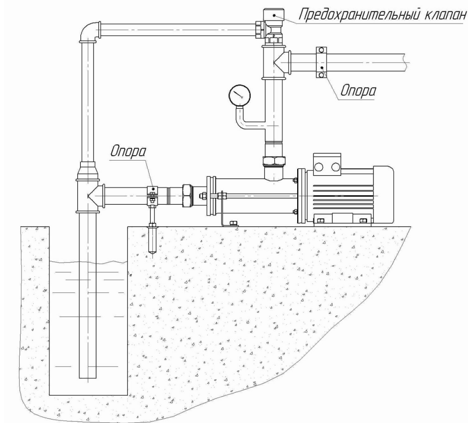
Рисунок 8 – Установка опор и крепления для труб.
