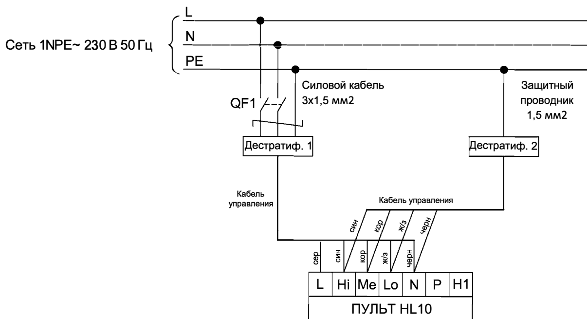
Рисунок 3. Схема подключения более двух дестратификаторов к одному пульту управления НЛ10
